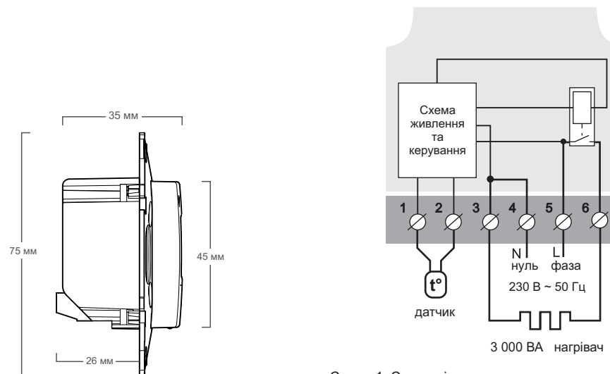
Схема 1. Схема підключення та спрощена внутрішня схема
